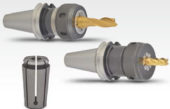
P.180 OZ/TG100 Collet Chuck 重切削筒夾本體
