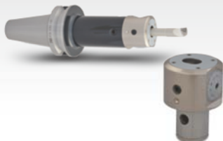
P.108 ABJ Modular Micro Boring Holder/Head 小徑微調搪刀桿 / 刀頭
