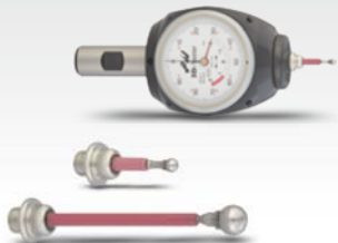
P.207 3D Sensor-Haimer 萬向尋邊器
